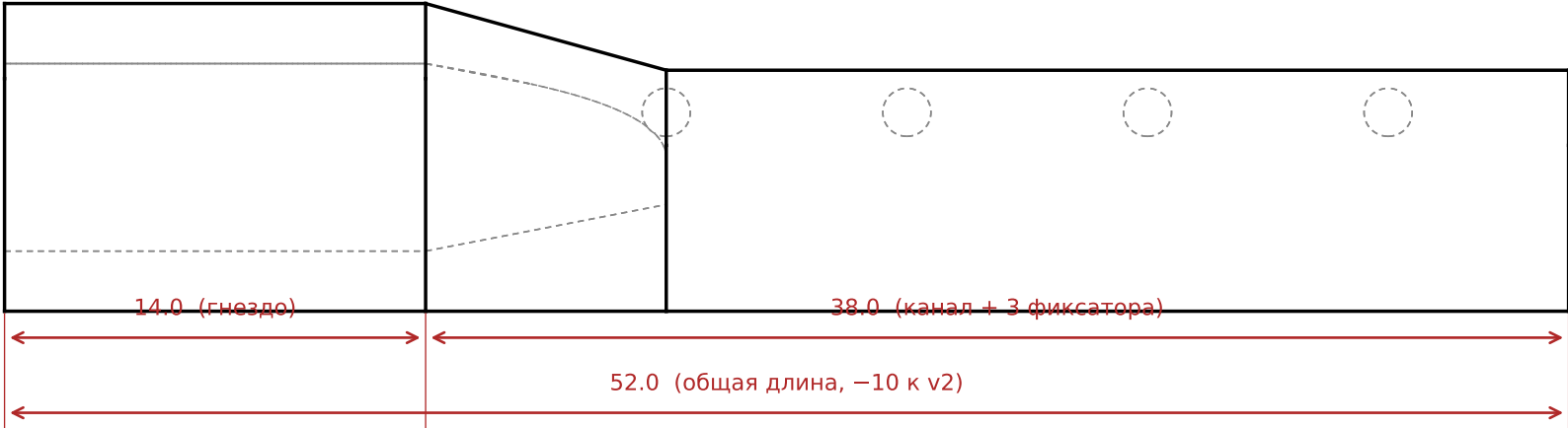
Вид сбоку (профиль X-Z)
